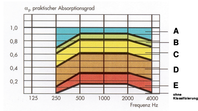
Abb. 19: Schallabsorptionsklassen A bis E gemäß DIN EN ISO 11654
